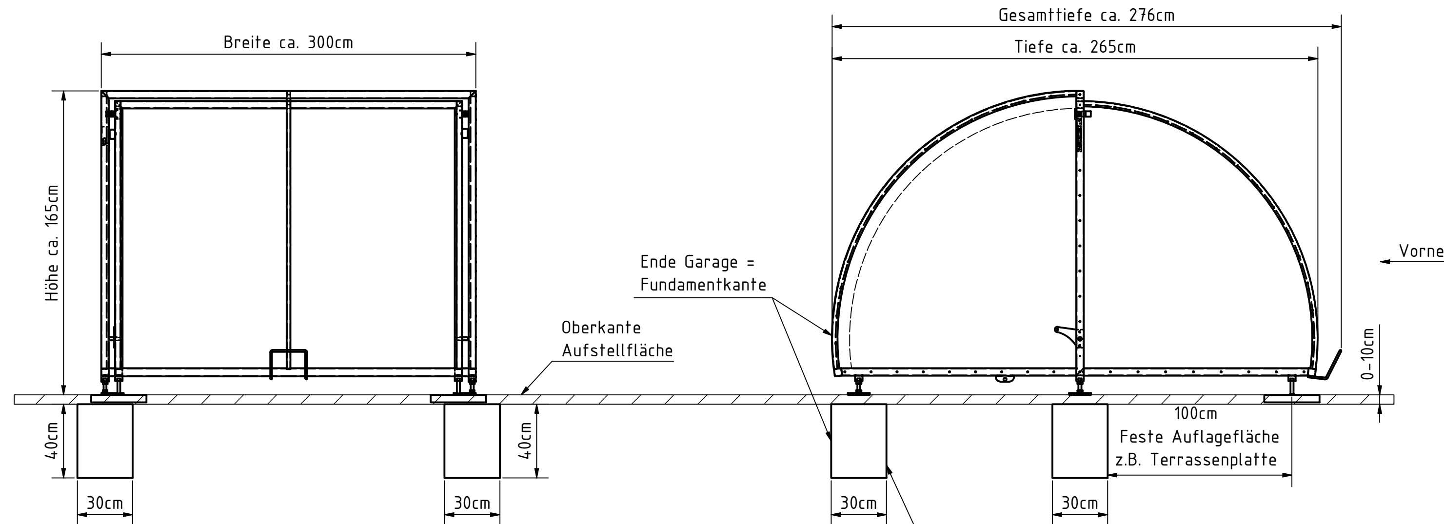
Vorderansicht
